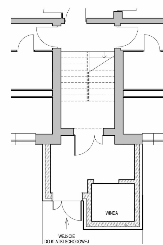
RZUT SKALA 1:100
