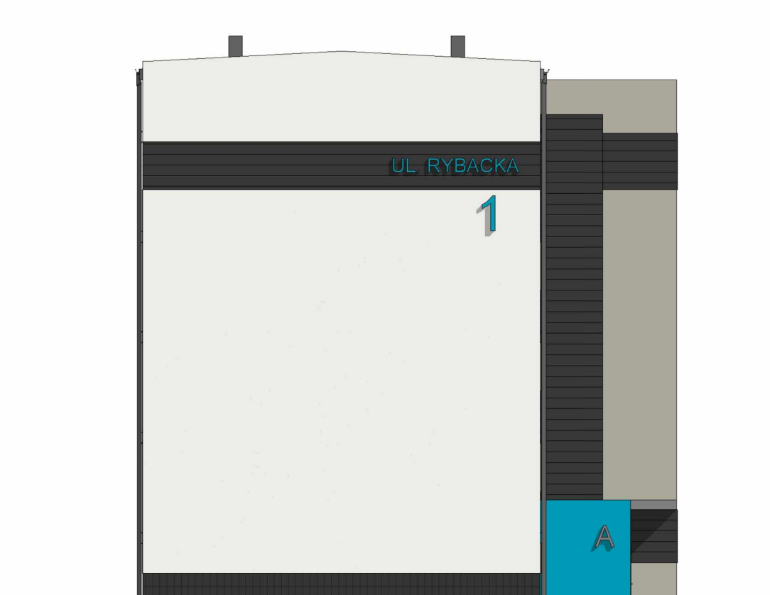
ELEWACJA POŁUDNIOWA
